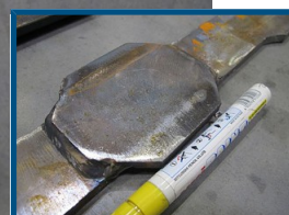
Figuur 10: vermoeingsscheur geïnitieerd aan een onderflens
